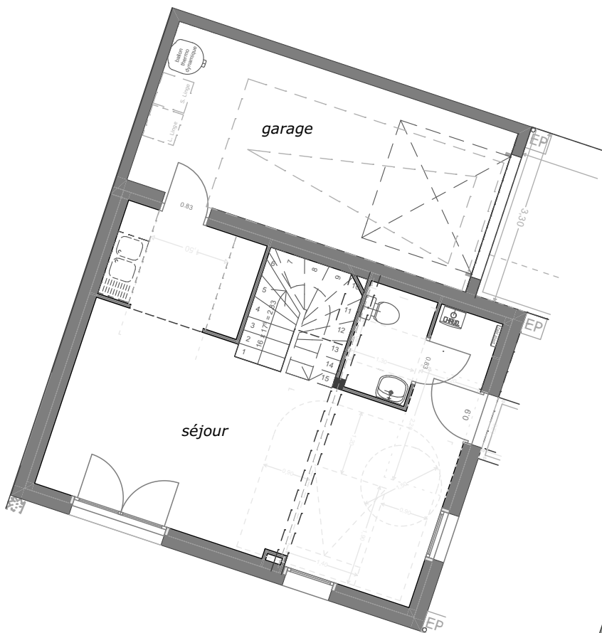
PLAN ETAGE
