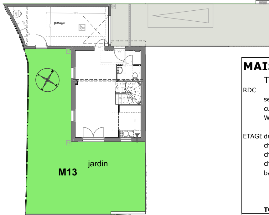
PLAN JARDIN
