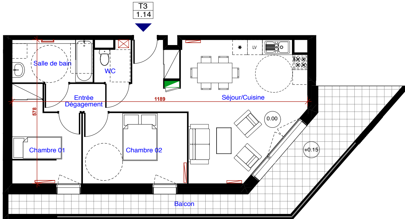
PLAN LOGEMENT ACCESSIBLE
