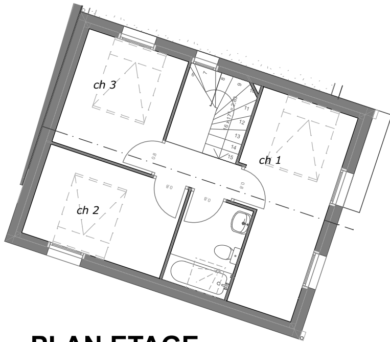
PLAN ETAGE
