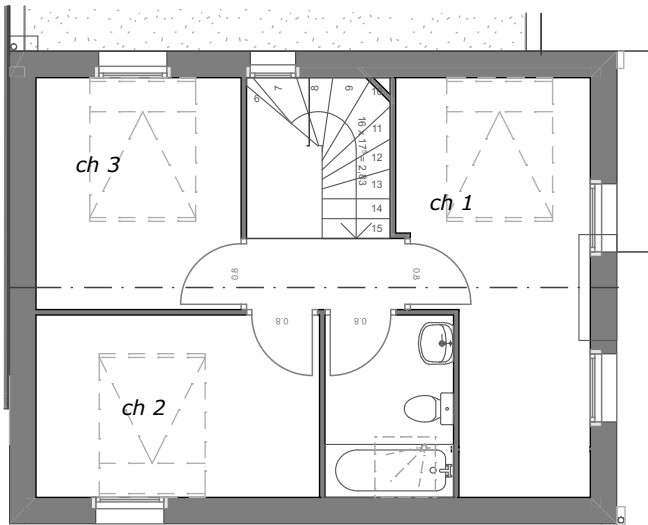
PLAN ETAGE
