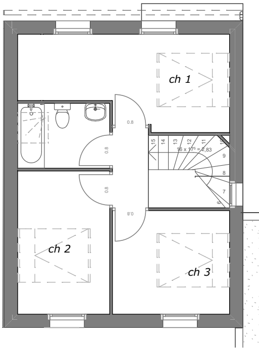
PLAN ETAGE
