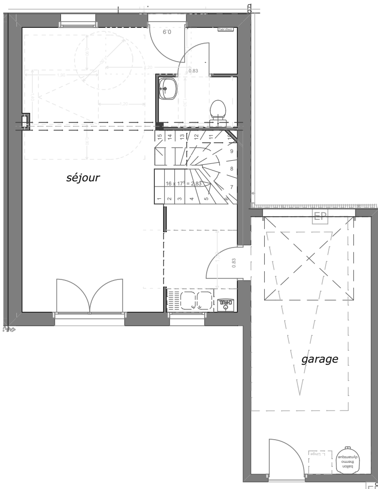
PLAN RDC
