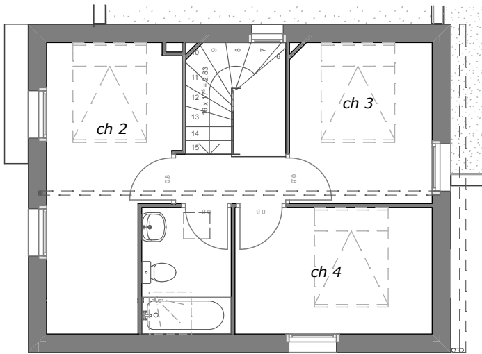
PLAN ETAGE
