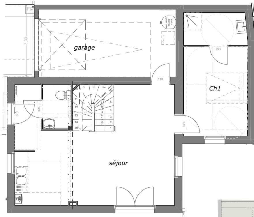
PLAN RDC
